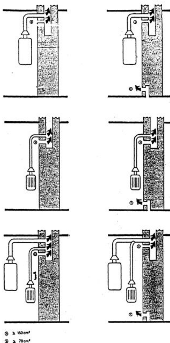
Slika 9 - Primer odvoda produkata sagorevanja od aparata sa osiguračem strujanja preko odvodnog kanala iz člana 127 ovog pravilnika
