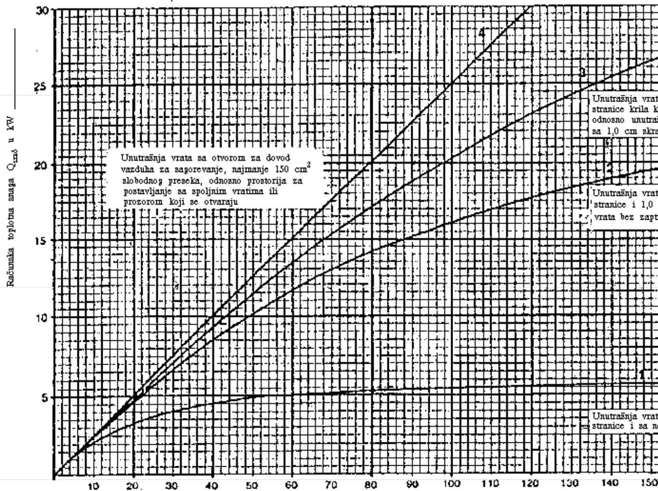
Dijagram 1 - Određivanje računске toplotne snage Q_{izm}
