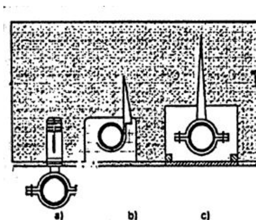
Slika 3 - Primeri postavljanja gasovoda
