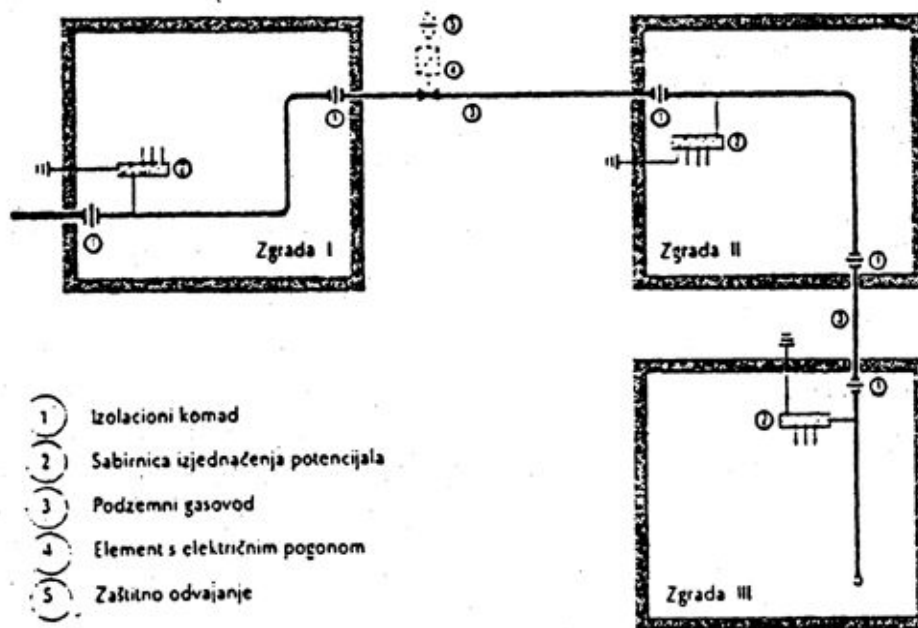
Slika 2 - Primer ugradnje izolacionih komada
