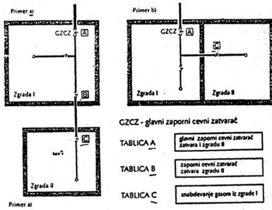
Slika 1 - Primeri ugradnje i označavanja zapornih cevni zatvarača
