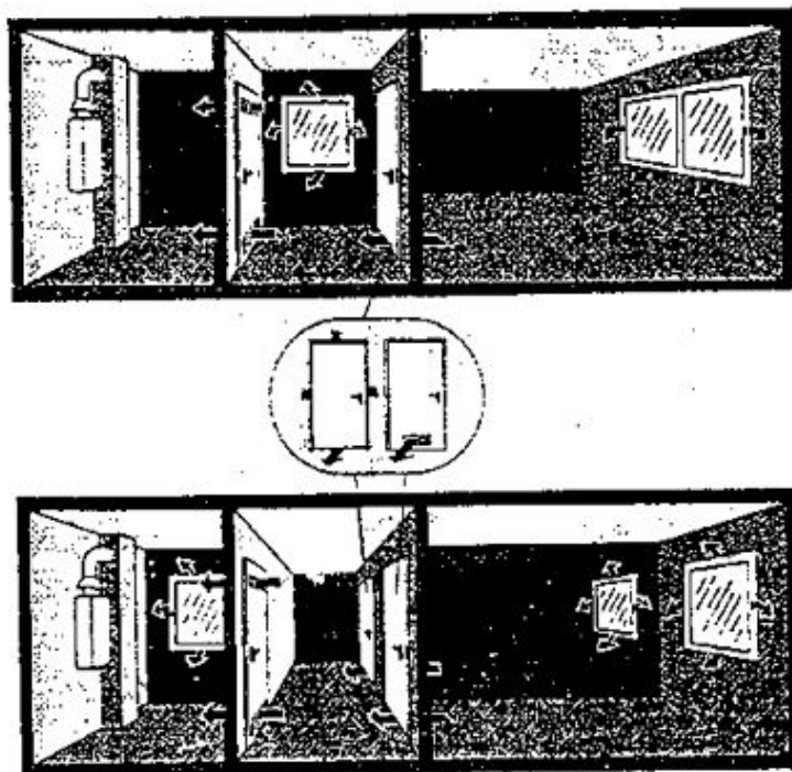
Posredno povezivanje dovoda vazduha za sagorevanje
