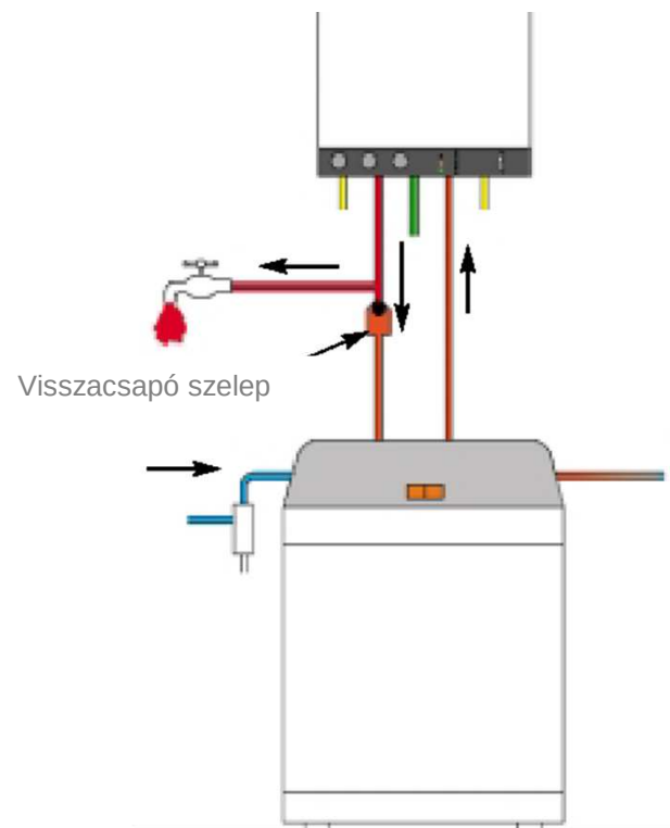
Folyamatos HMV elvétel a tárolóból és a kazánból
