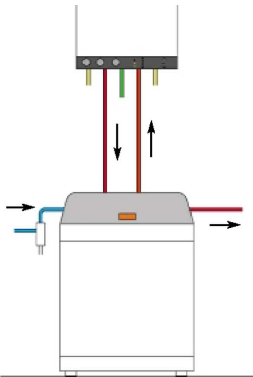
Folyamatos HMV elvétel a tárolóból
